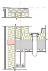
1. PARAPET
